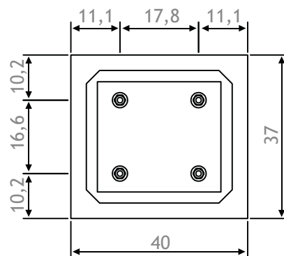
Vista superior anclas
