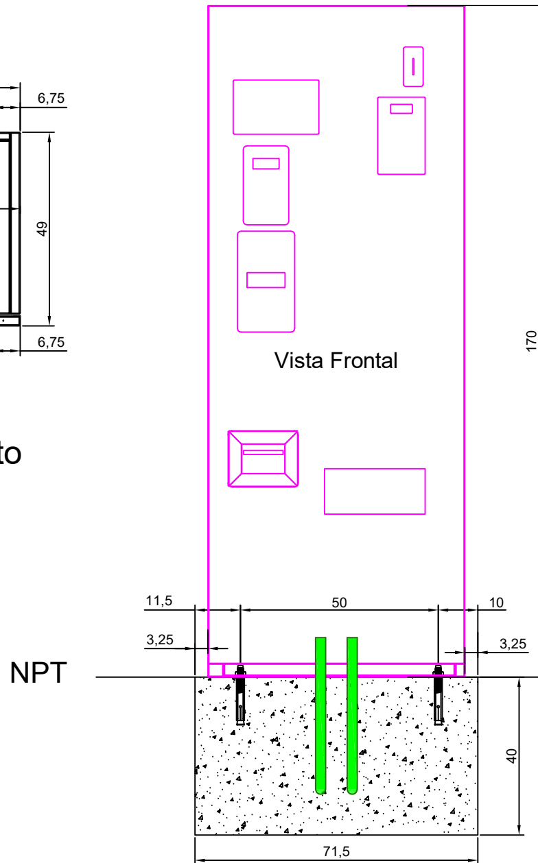
Frente Modulo
