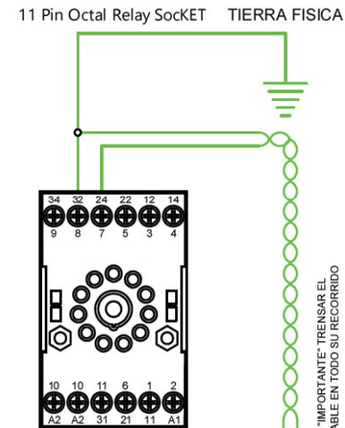
SENSOR DE MASA BEA FAMILIA MATRIX-2-S
