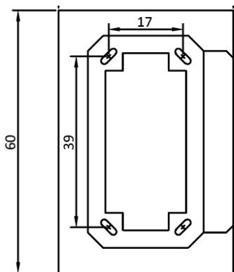
Vista superior anclas
